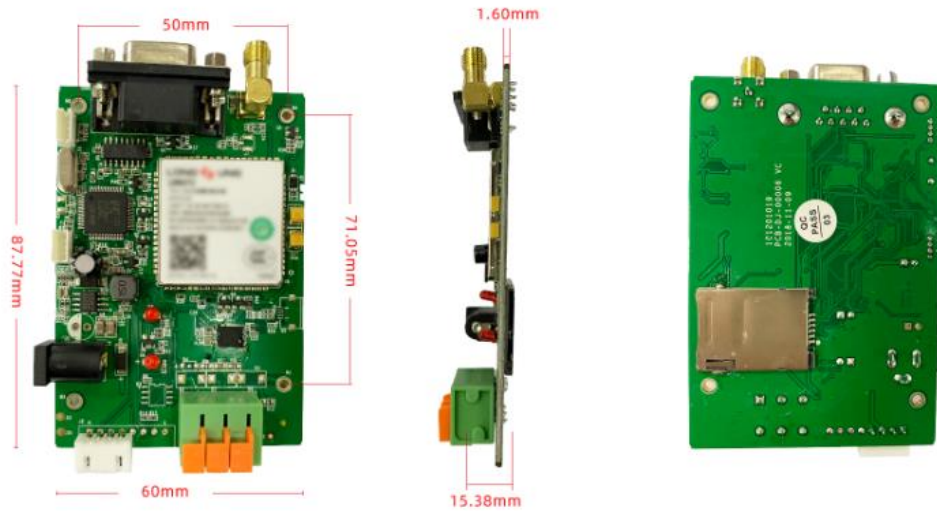
模板尺寸：87.77*60*15.38mm
