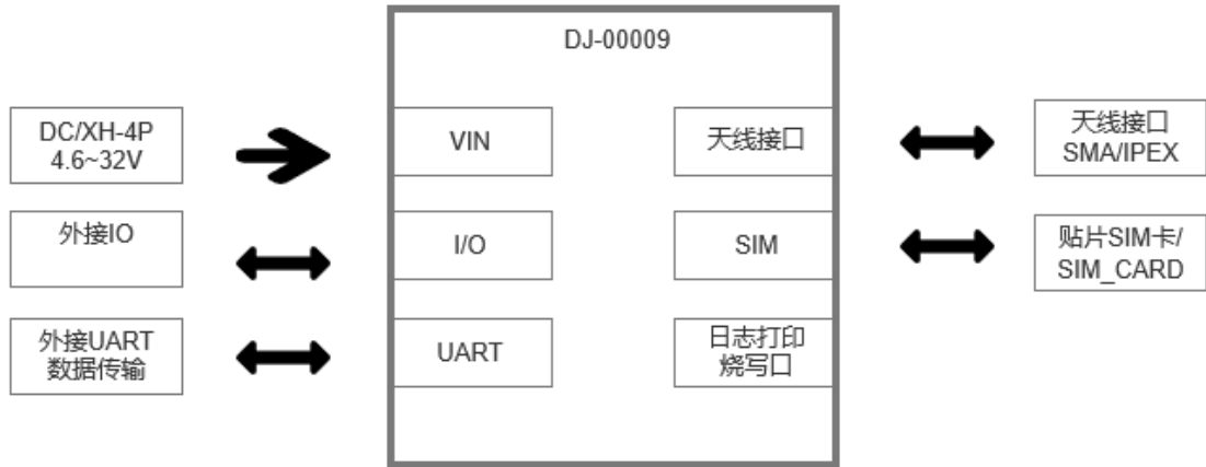
模块外围参考电路
